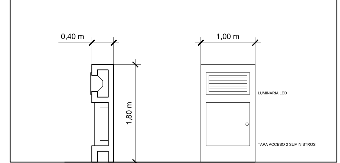
DETALLE MONOLITO LUMINARIAS / ACOMETIDAS
