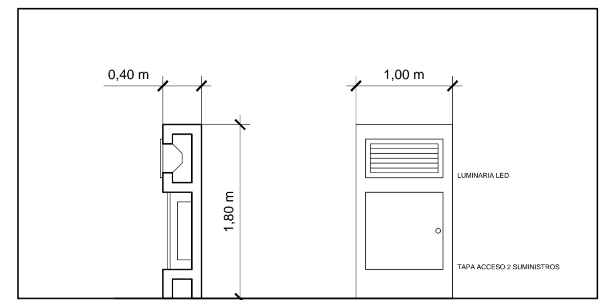
DETALLE MONOLITO LUMINARIAS / ACOMETIDAS
